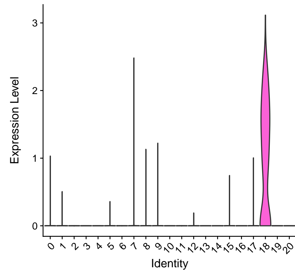
FCRL1
