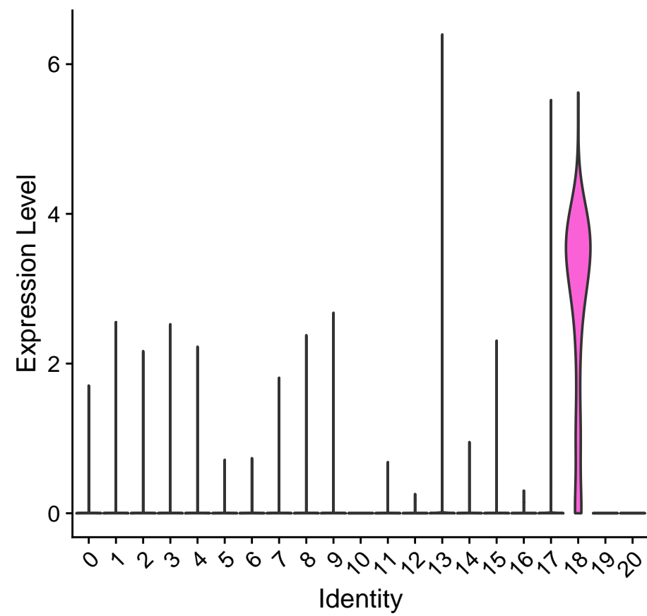
TCL1A
