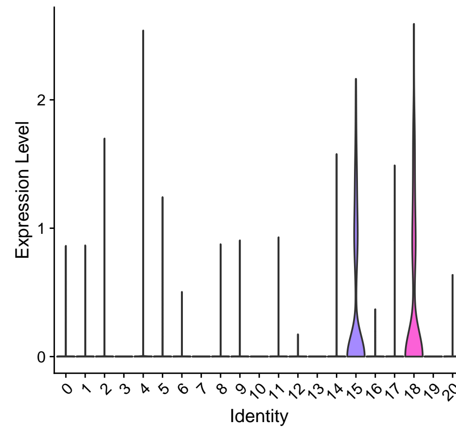
SLAMF1
