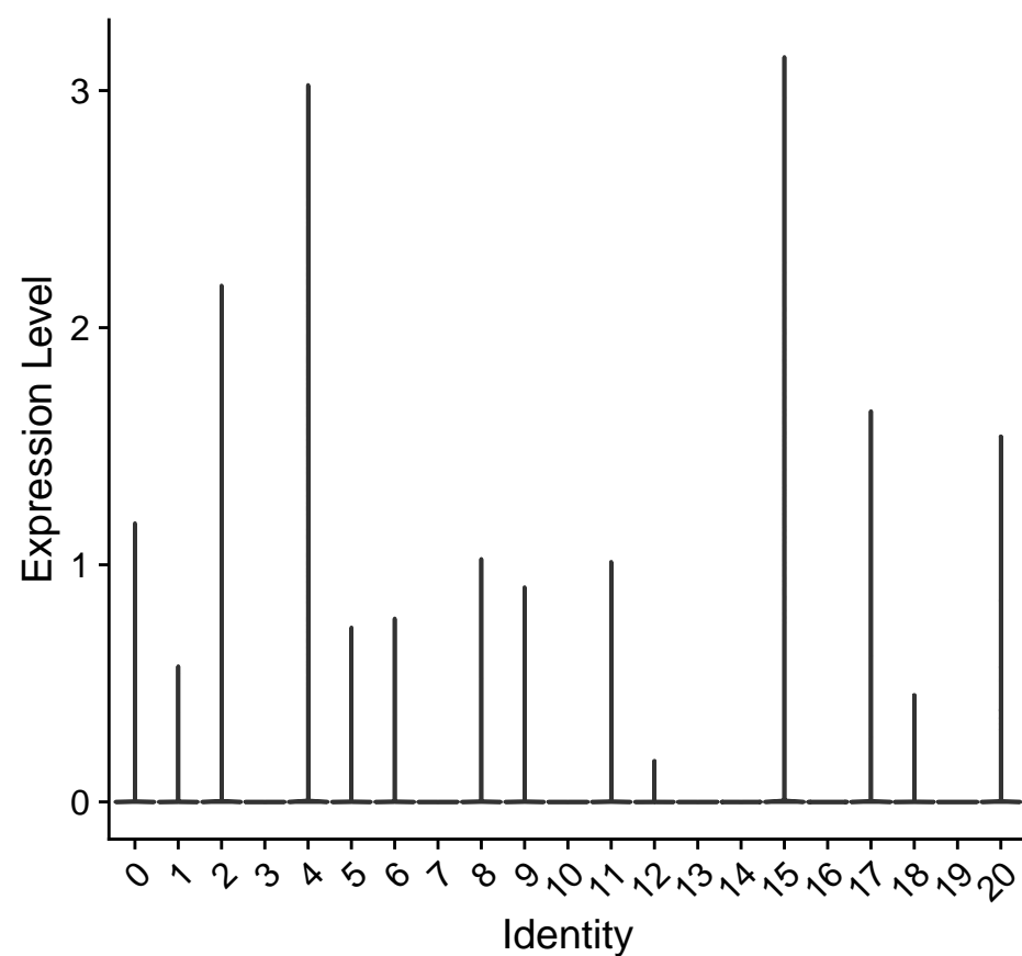
CXCR6
