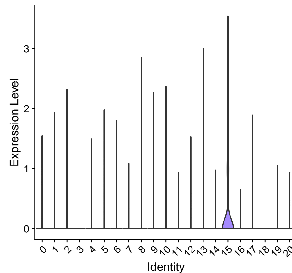
LAG3
