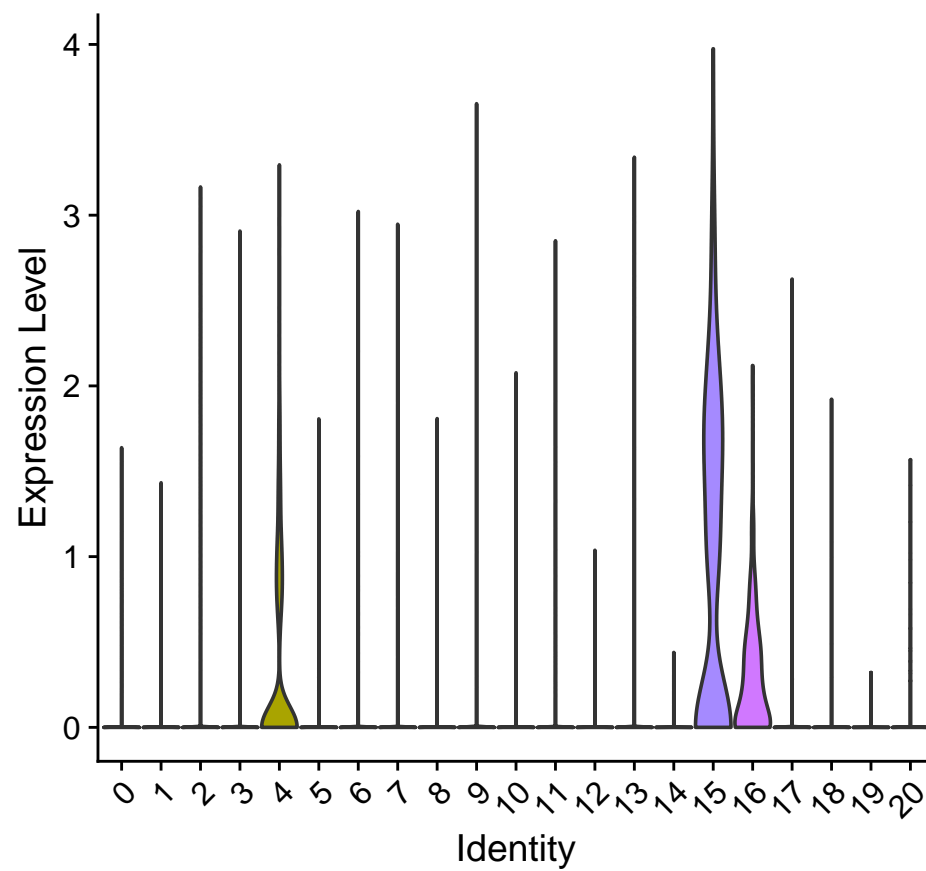
GRAP2
