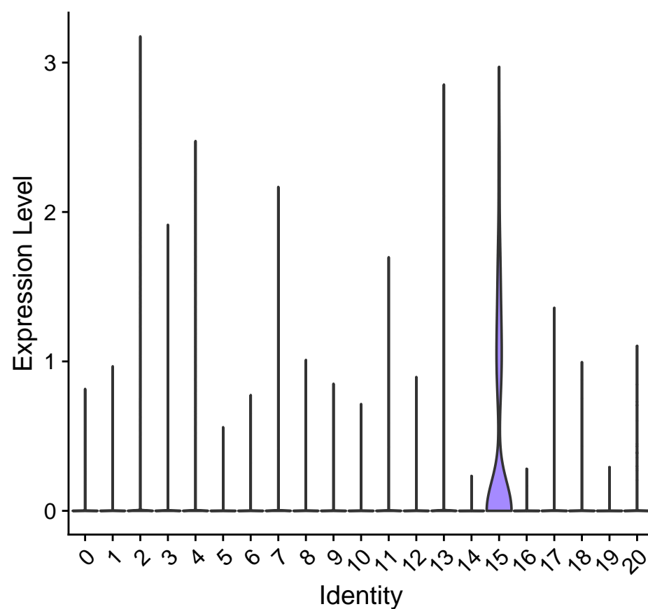
KLRG1
