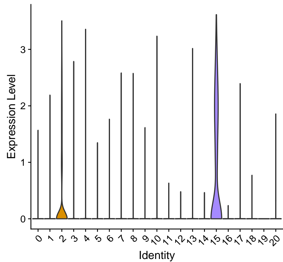
CD8A
