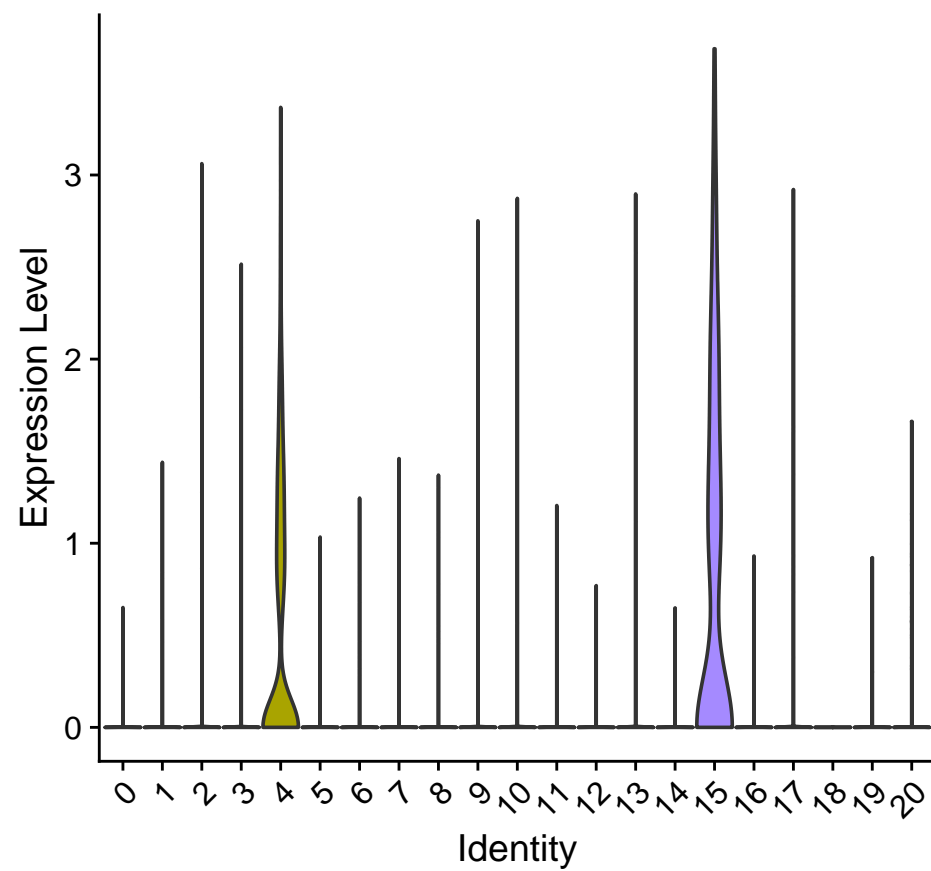
CD40LG
